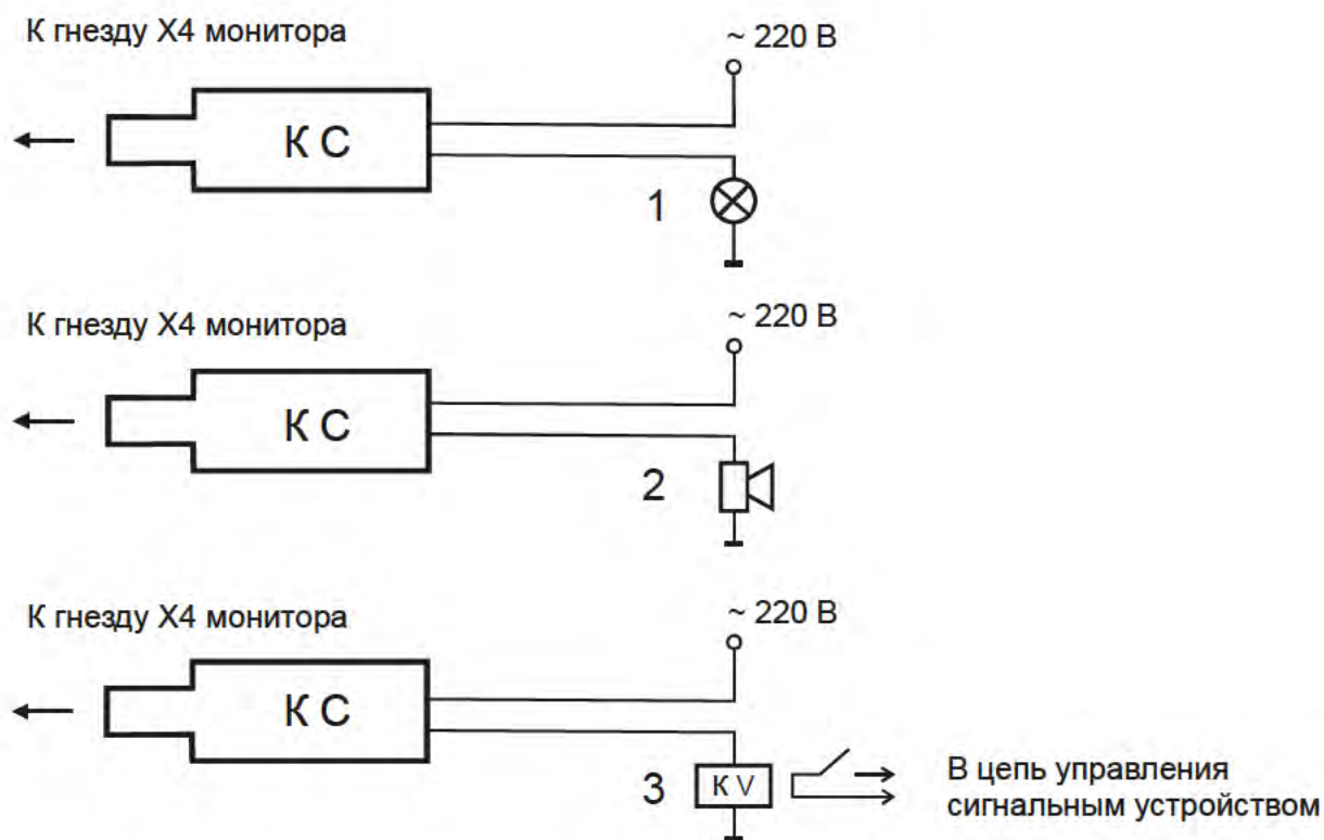
Рисунок 11 - внешний вид и варианты схем подключения контакта сигнального КС:
