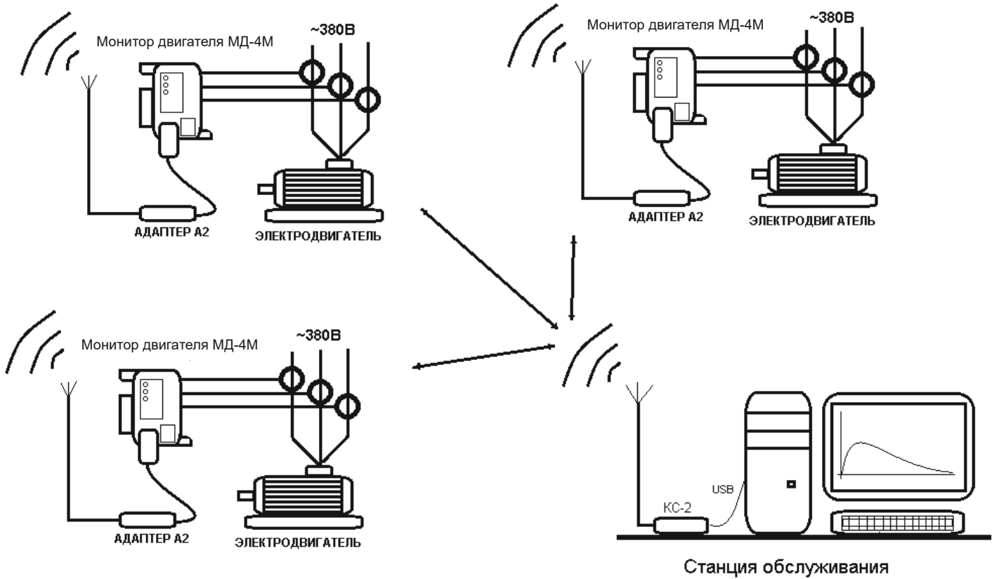
Рисунок 28 – схема организации связи в сети беспроводного доступа
