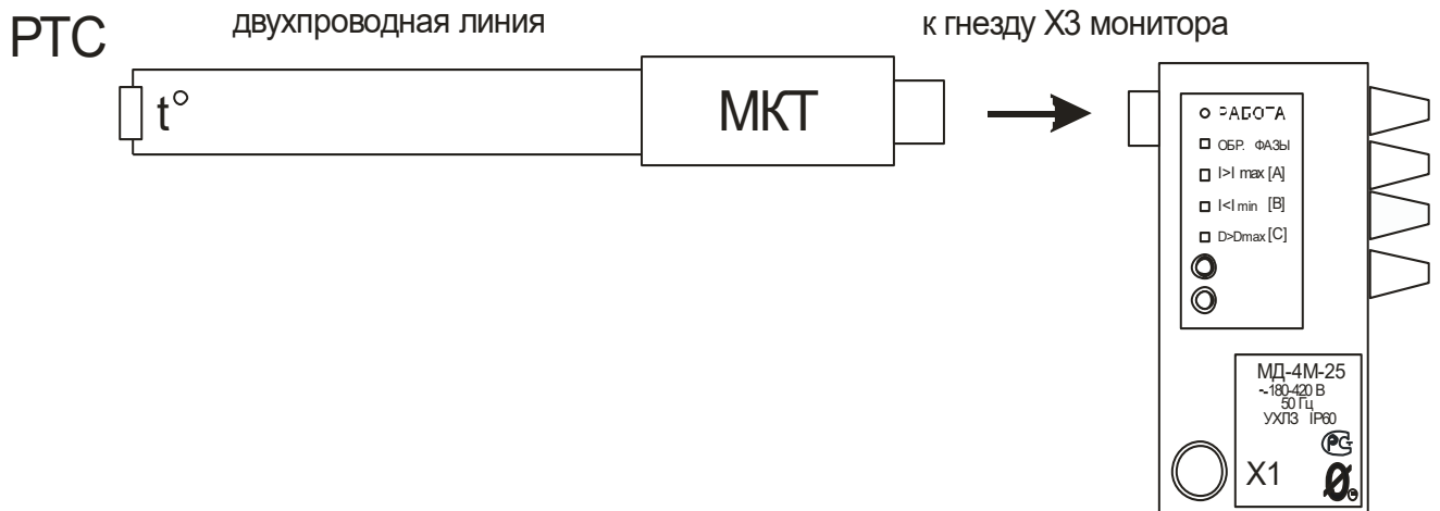
Рисунок 29 – подключение модуля контроля температуры
