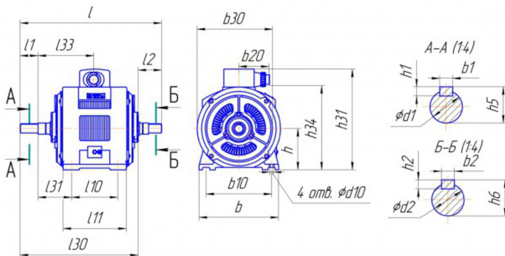
Электродвигатели серии 4АЛ. IM 1001, IM 1002.
