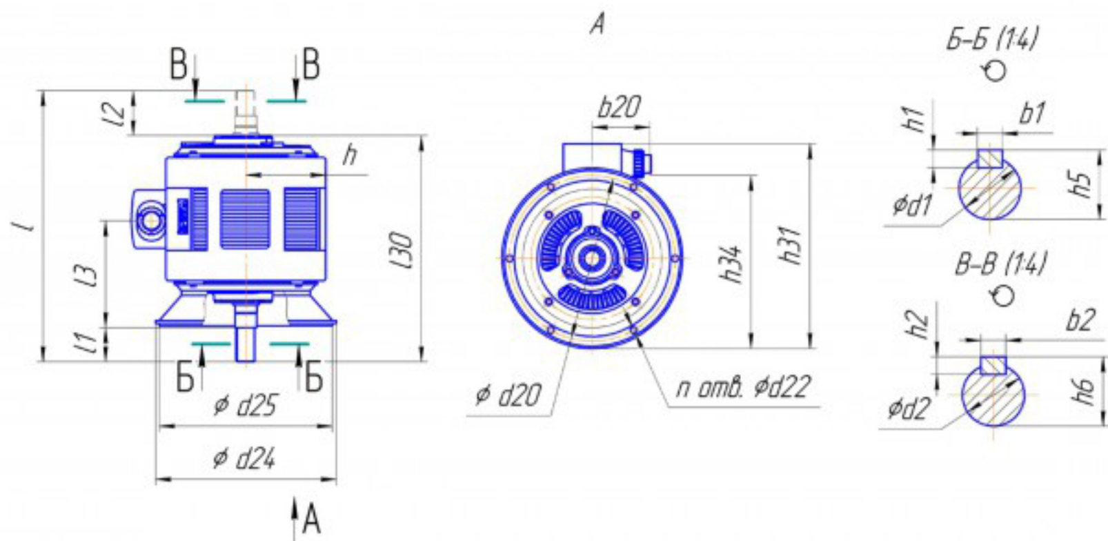
Электродвигатели серии 4АЛ. IM 3001, IM 3002.
