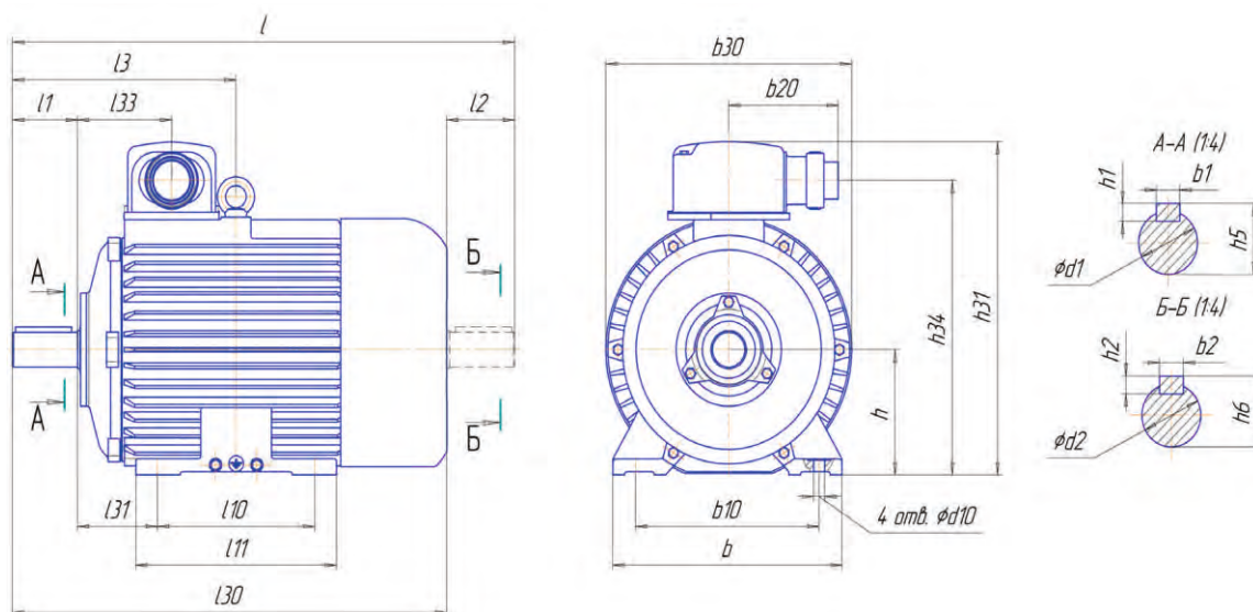
Электродвигатели серии 5AM. 5AM-200, 5AM-250. IM 1001, IM 1002. Низковольтные.
