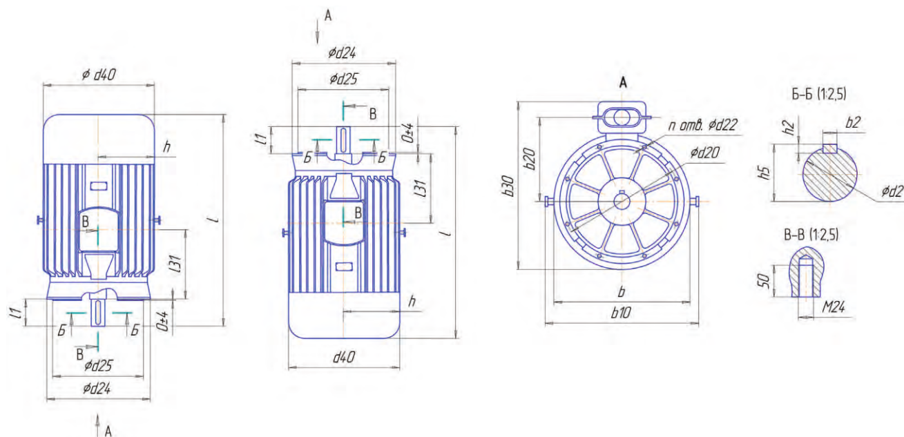
Электродвигатели серии 5AM. 5AM-355. IM 3011, IM 3031. Низковольтные
