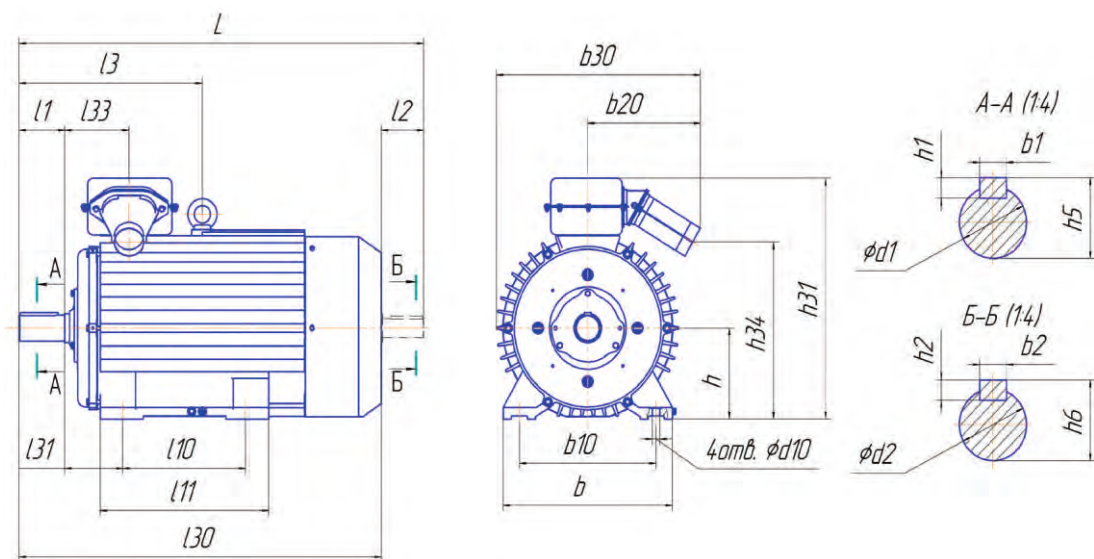
Электродвигатели серии 5AM. 5AM-315. IM 1001, IM 1002. Низковольтные.
