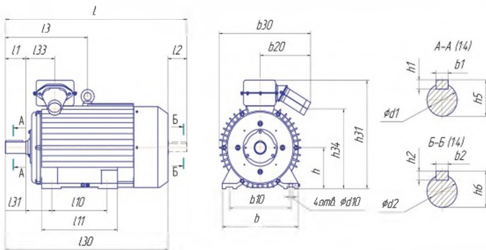
Электродвигатели серии 5AM. 5AM-315. IM 1001, IM 1002. Низковольтные.
