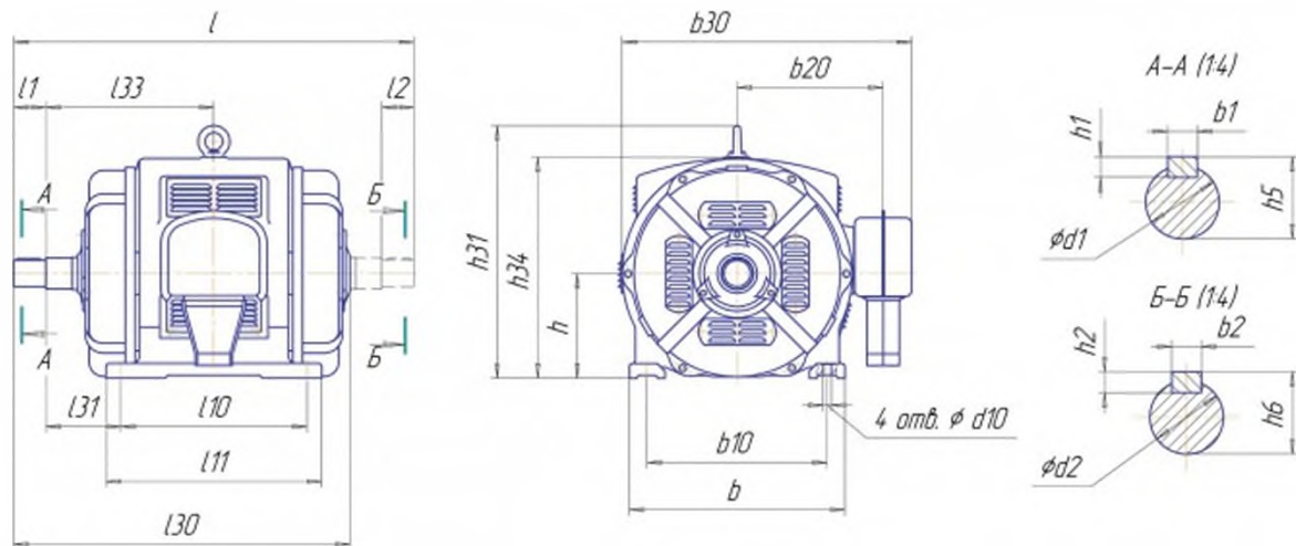
Электродвигатели серии А4. А4-355. IM 1001, IM 1002. Высоковольтные.
