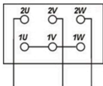
Схема соединения обмоток двигателей 6/4; 8/6 ( Y/Y/Y )
