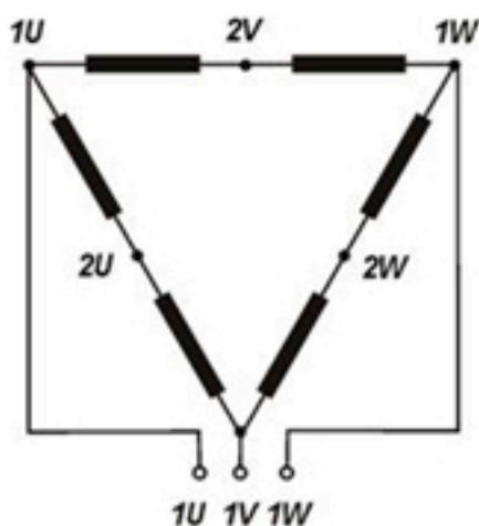
Схема соединения обмоток двигателей 4/2; 8/4 ( \Delta/Y/Y )
