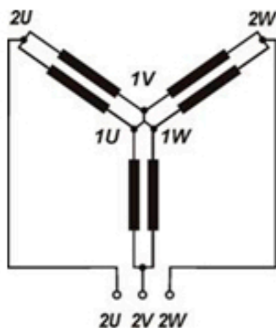
Схема соединения обмоток двигателей 4/2; 8/4 ( \Delta/Y/Y )
