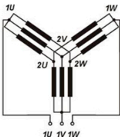
Схема соединения обмоток двигателей 6/4; 8/6 ( Y/Y/Y )
