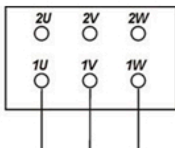
Схема соединения обмоток двигателей 6/4; 8/6 ( Y/Y/Y )
