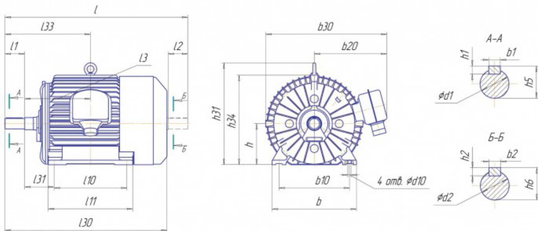
Электродвигатели серии АО2-9. IM 1001, IM 1002. Многоскоростные.
