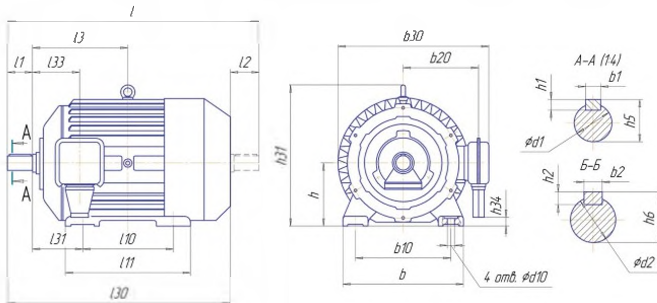
Электродвигатели серии АОЗ. АОЗ-400 IM 1001. Низковольтные.
