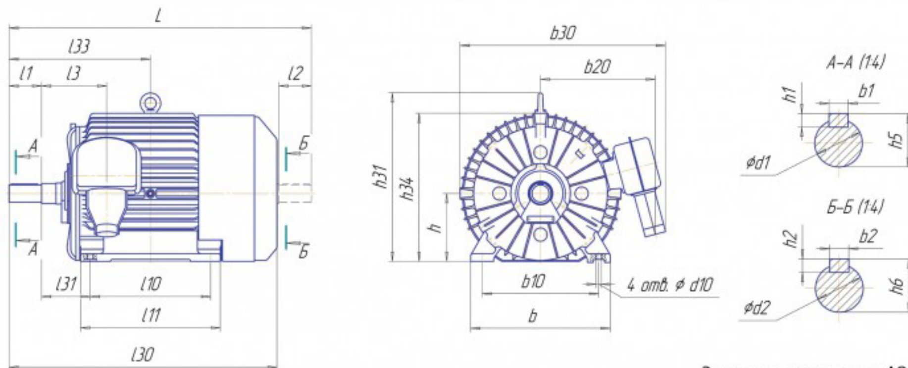
Электродвигатели серии АО4. АО4-355 IM 1001, IM 1002. Высоковольтные.
