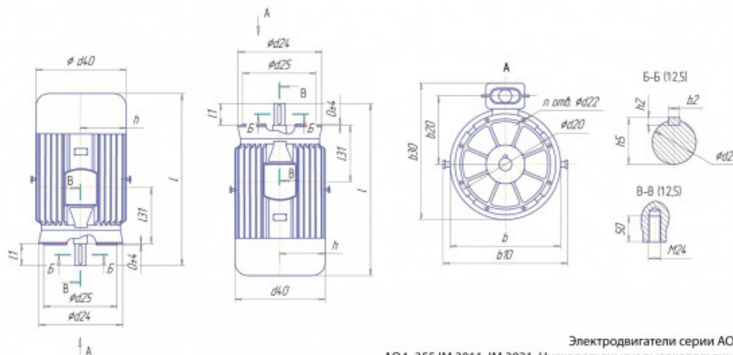
Электродвигатели серии А04. А04-355 IM 3031. Низковольтные.
