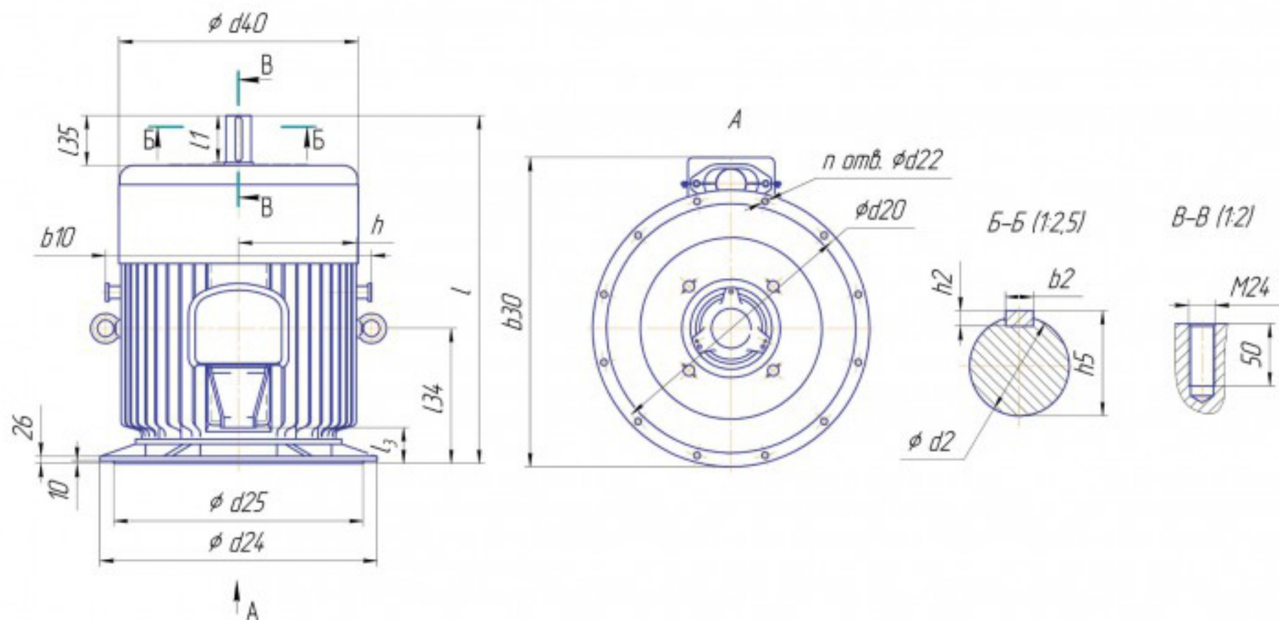
Электродвигатели серии А04. А04 IM 3132 низковольтные специального исполнения с пониженной мощностью SAD
