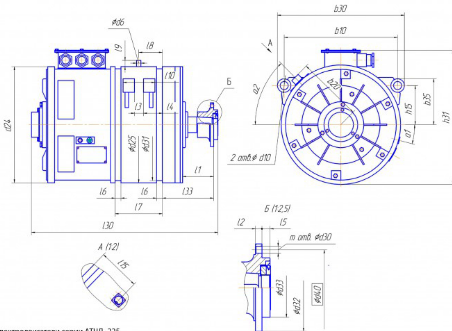
Электродвигатели серии АТЧД-225.
