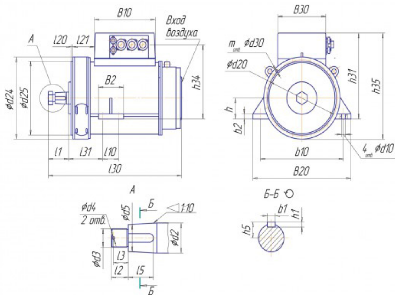
Генераторы БГ-160 и БГ-200 общепромышленного исполнения (исполнение на 2 лапах)
