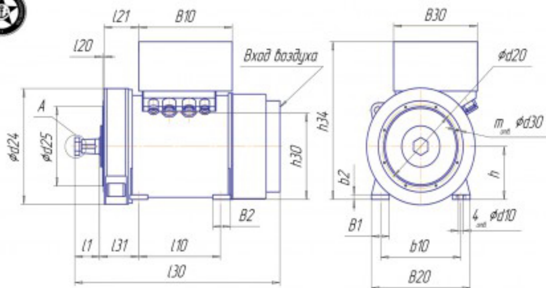
A(12,5) Вал генератора 16-30 кВт
