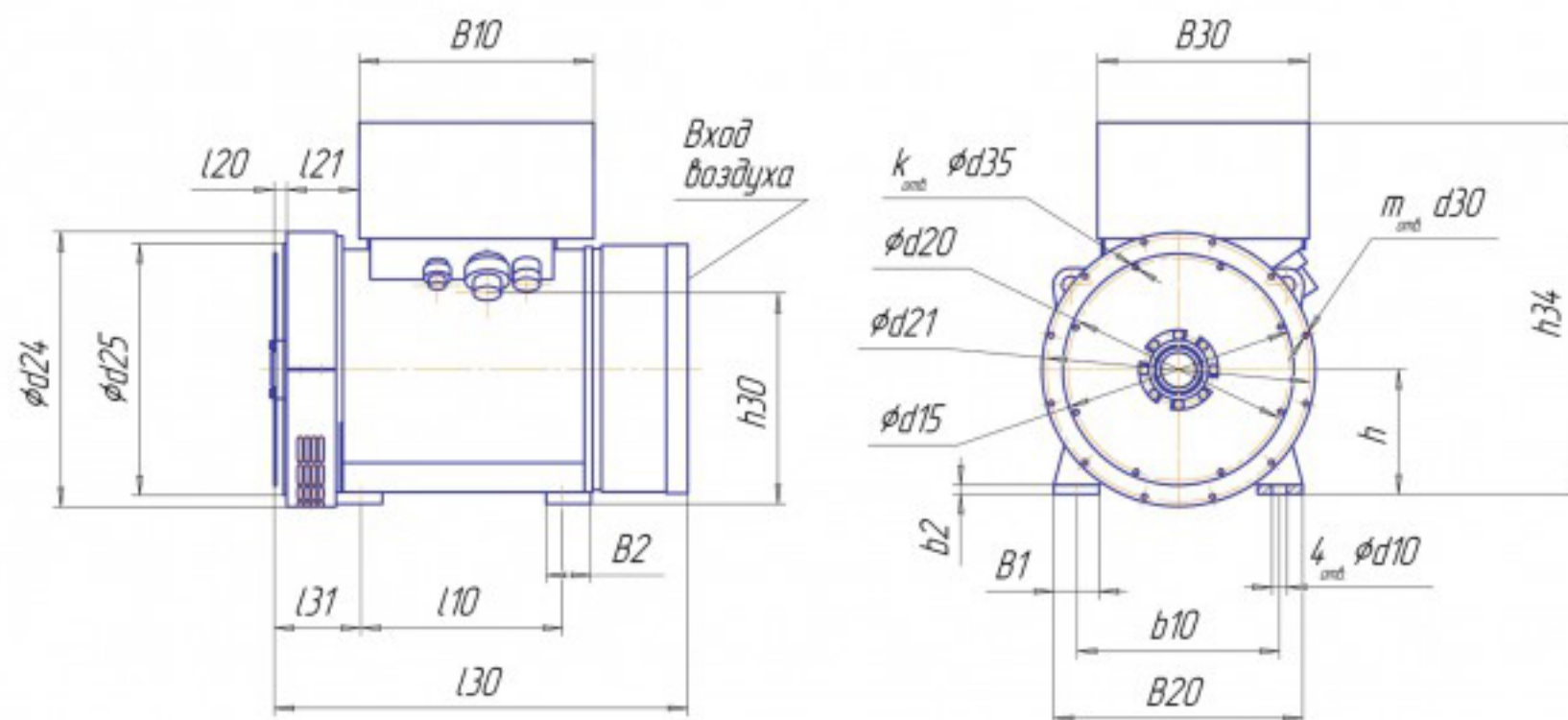
Генератор серии БГО общепромышленного исполнения.
