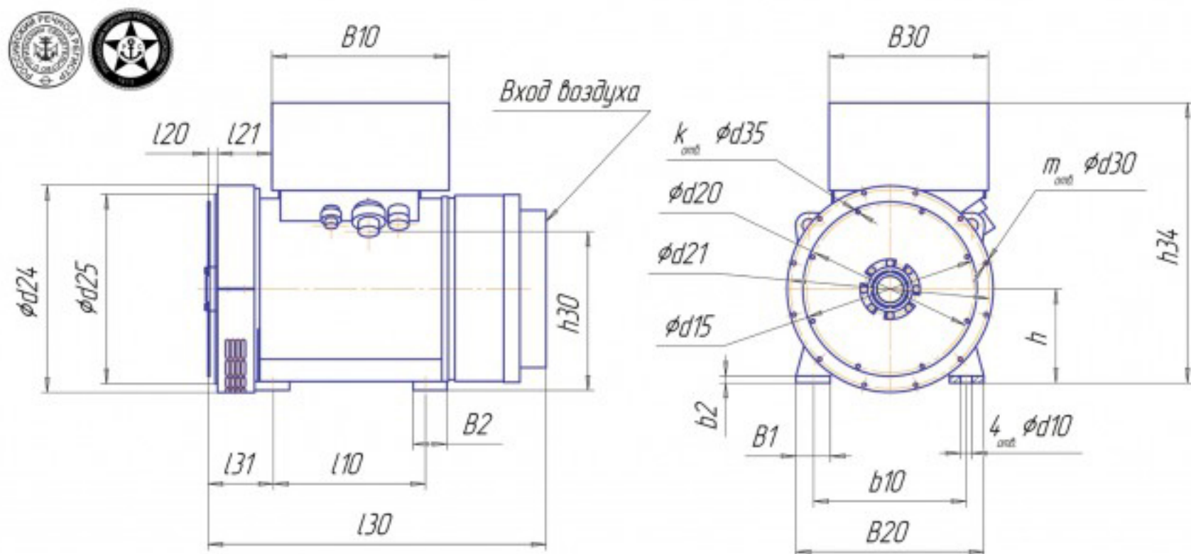
Генератор серии БГО судового исполнения.
