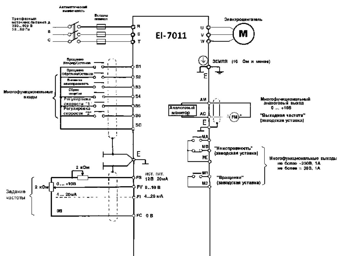
Рис. 9. Схема подключения.
