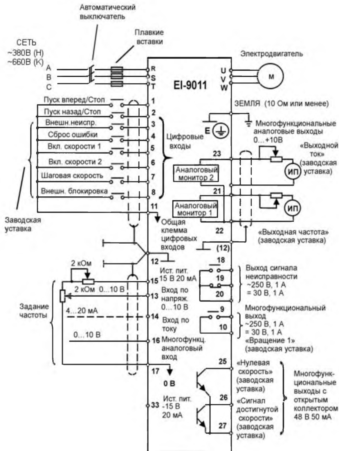
Рис. 4. Схема подсоединения
