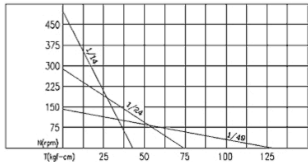
Коллекторный двигатель постоянного тока, 24В
