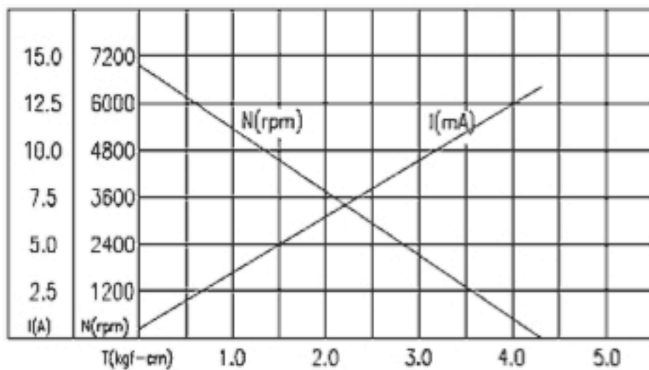
Коллекторный двигатель постоянного тока, 24В
