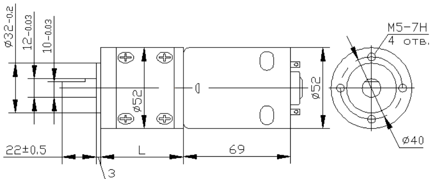
Габаритные и присоединительные размеры мотор-редуктора IG-52GM
