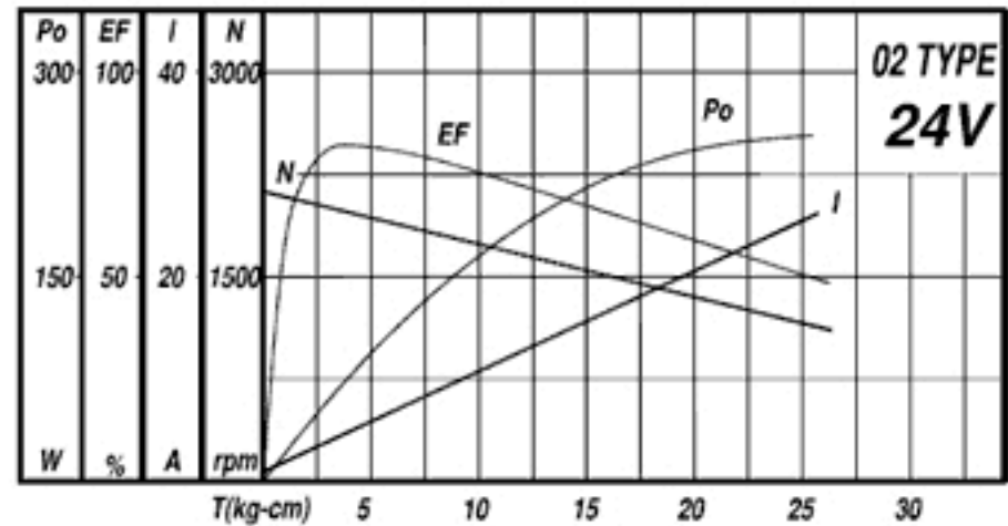
Коллекторный двигатель постоянного тока
