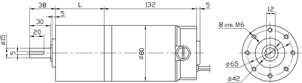
Габаритные и присоединительные размеры мотор-редуктора РТС7152
